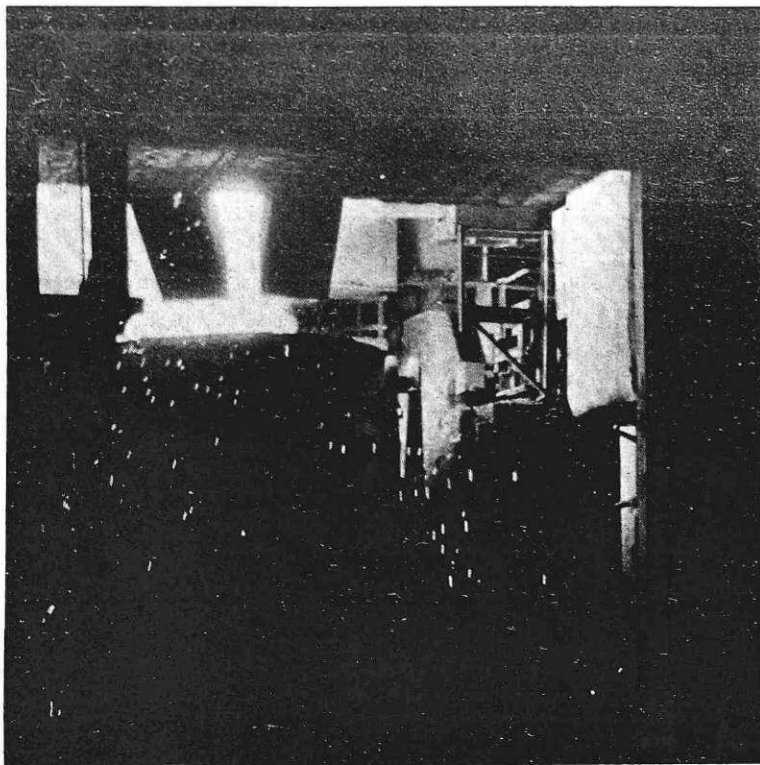
Sarž na elektro peči v Jeklarni 2 (foto: Irena Kučina)
