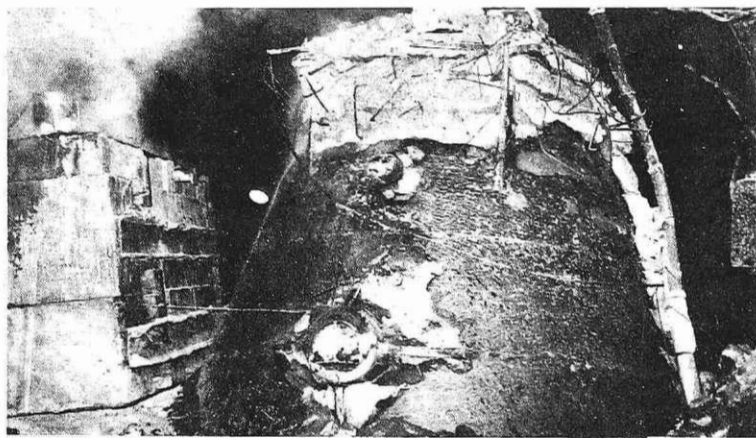
Ponovca, vlita iz jekla zadnjega sarža tretje SM peči (foto: S. Kokalj)
