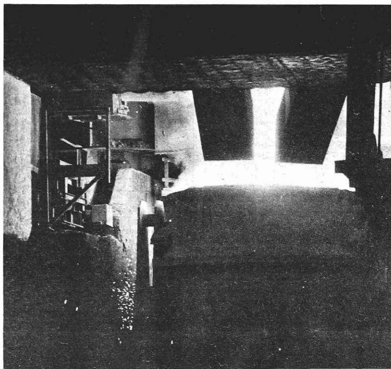
Prebod na elektro peči v Jeklarni 2 (foto: Irena Kučina)
