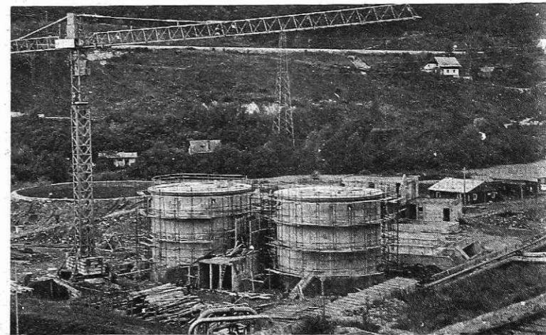
Mestna biološko čistilna naprava za komunalne odplake in odplake iz Železarnice (foto: Silvo Kokalj)
