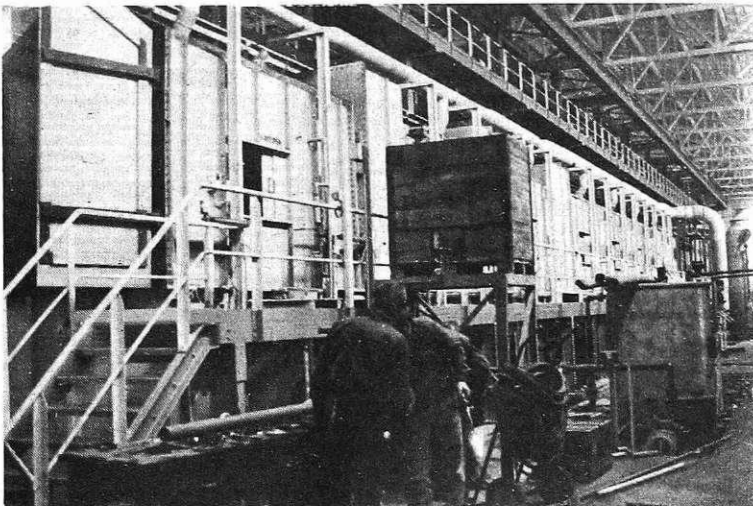
Nova lužilna linija v Hladni valjarni Jesenice (foto: I. Kučina)
