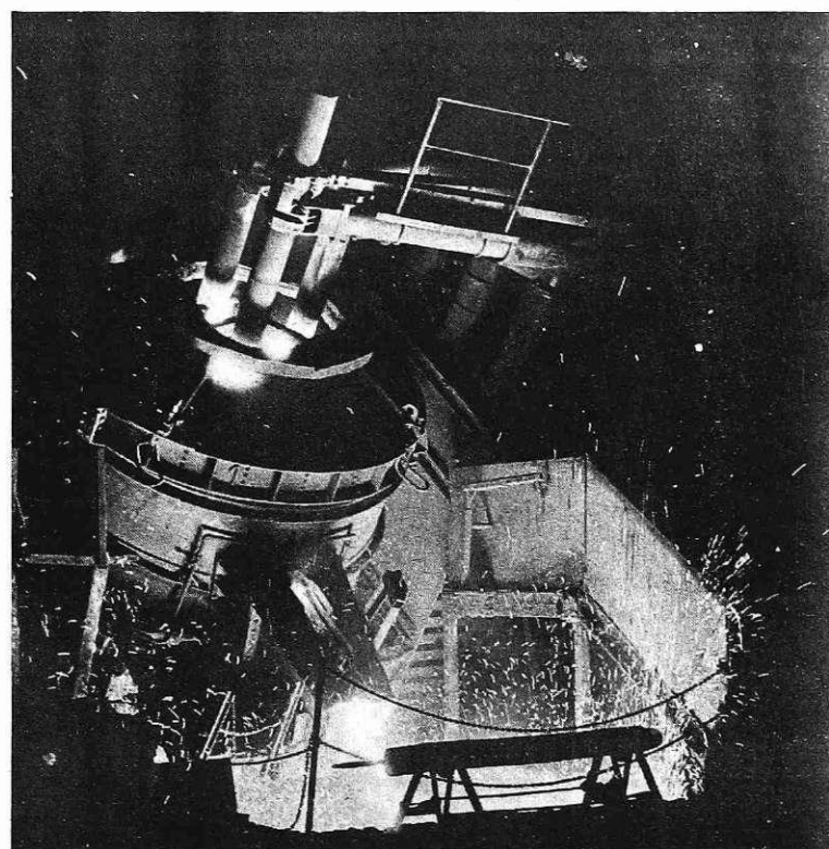
BBC elektro peč (foto: I. Kučina)
