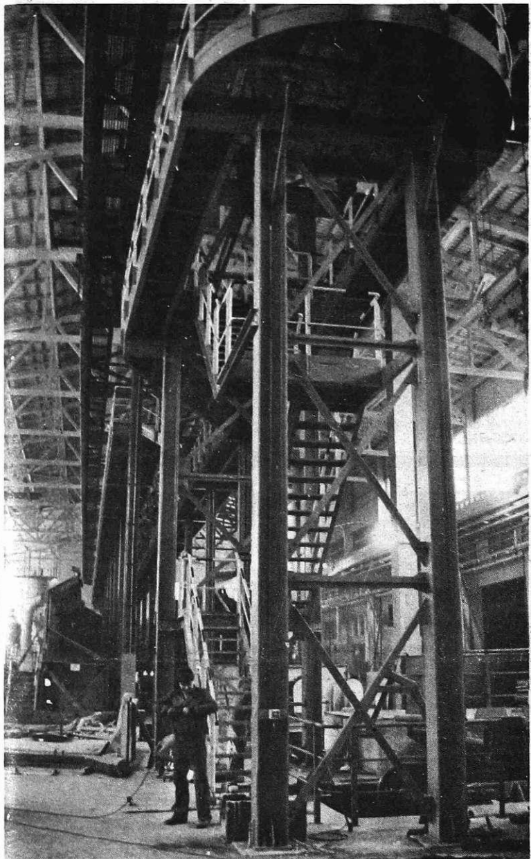
Montaža lužilne linije v Hladni valjarni Jesenice (foto: I. Kučina)
