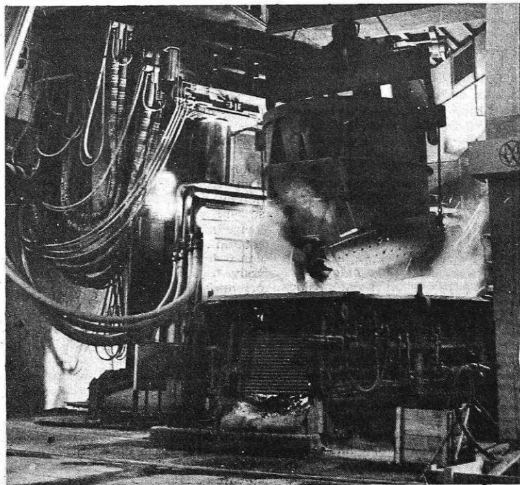
Zakladanje peči na Beli (foto: I. Kučina)
