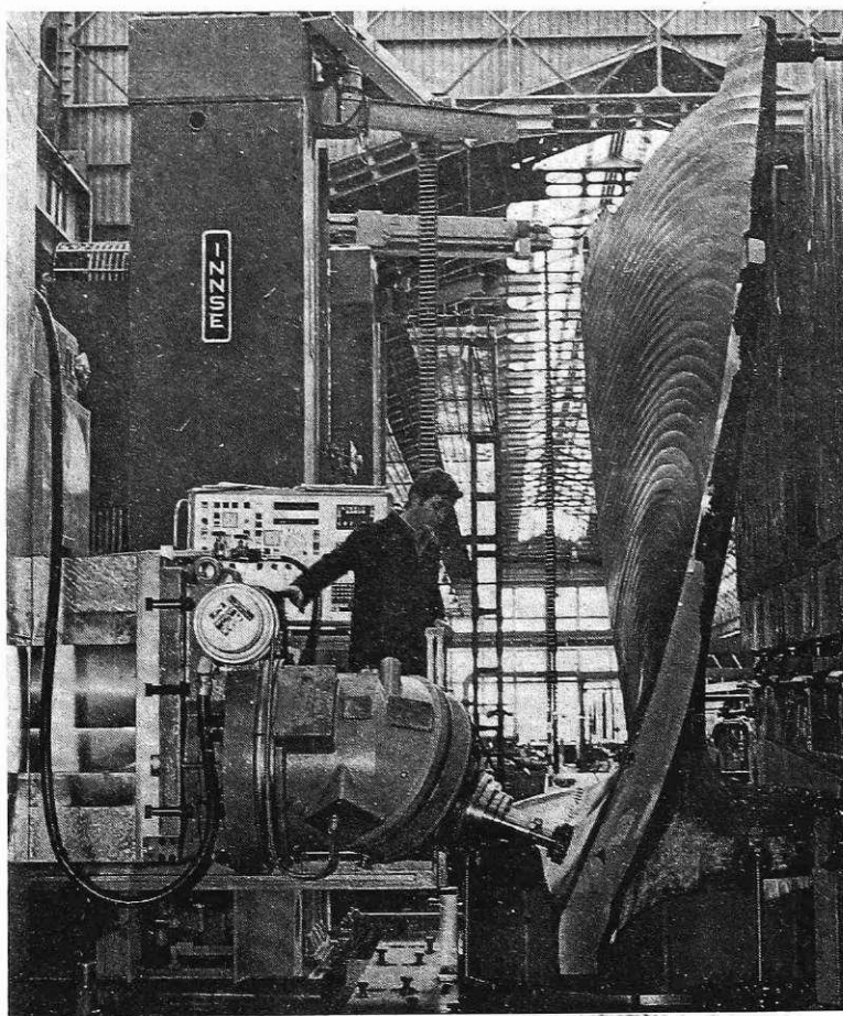
Lopatice Kaplanove turbine, ki jo izdelujejo v Innocenti
