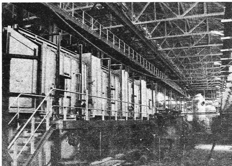
Montaža nove lužilne linije (foto: I. Kučina)
