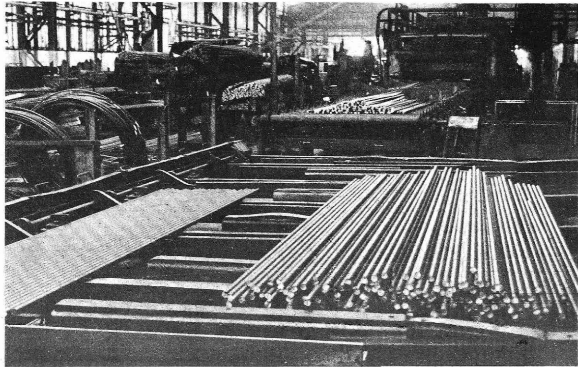
Jeklovlek (foto: Irena Kučina)
