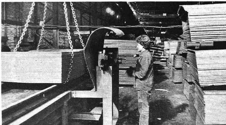
Tehtanje pločevine na liniji rezanja v Valjarni bluming (foto: I. Kučina)
