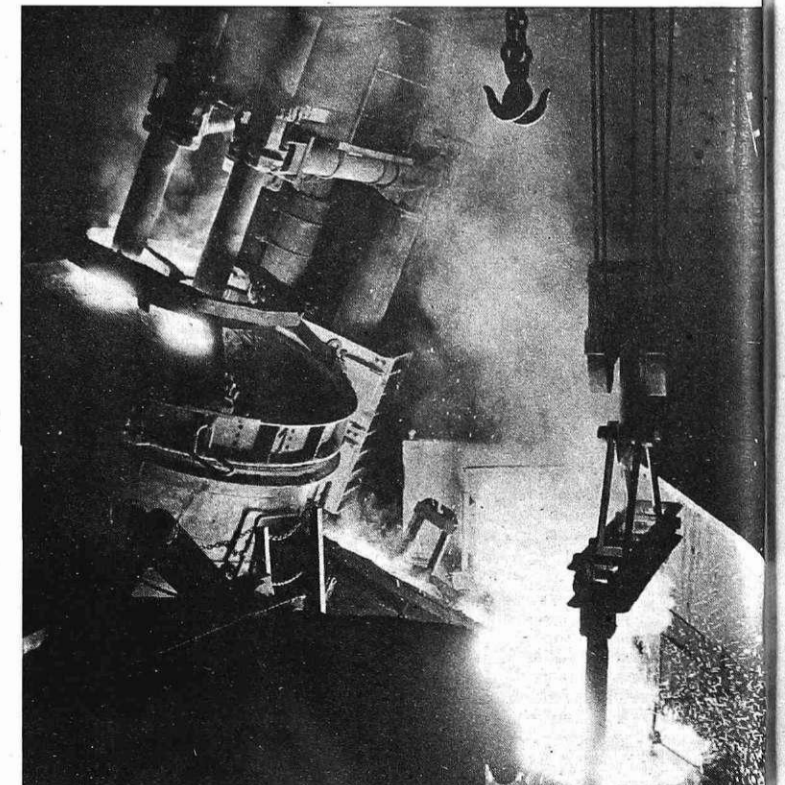
Prehod na BBC električni peči (foto I. Kučina)
