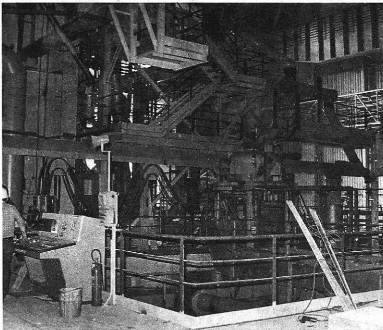
Testiranje naprave za vpihovanje kalcij-silicija (foto I. Kučina)
