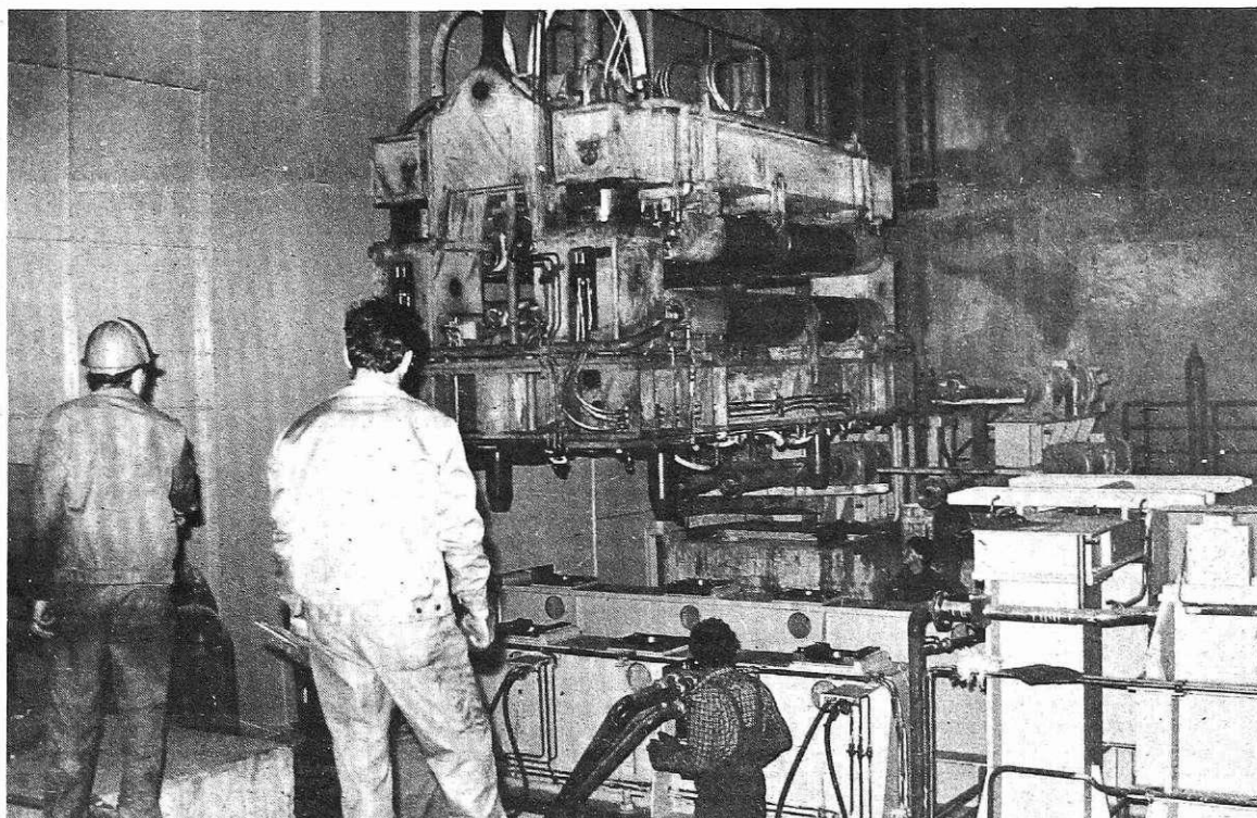
Montaža proge konti liva v Jeklarni 2 (foto I. Kučina)
