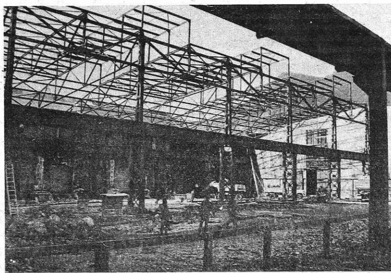
Gradnja Strojnih delavnic na Javorniku (foto I. Kučina)
