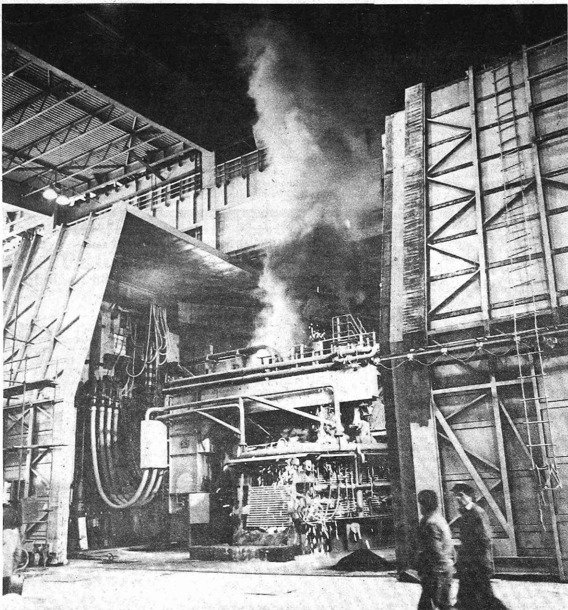
Nova elektropeč med obratovanjem (foto: I. Kučina)
