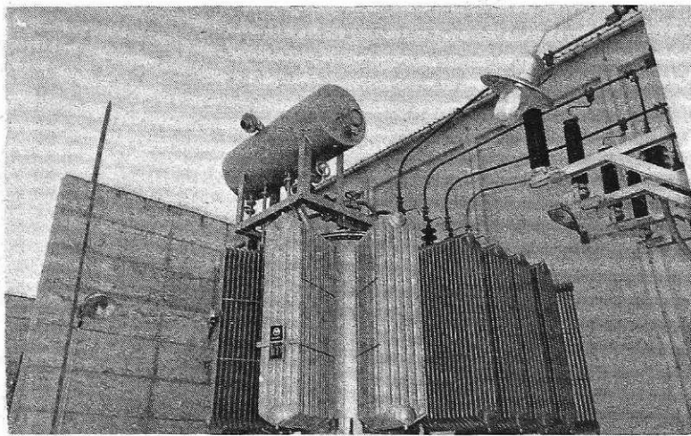
Transformator v RTP Jeklarna 2 (foto: B. Grce)
