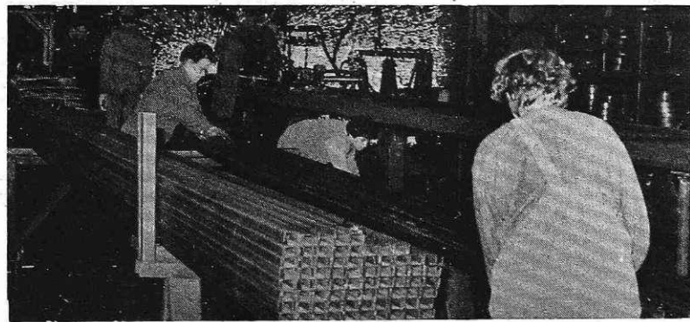
Izdelava hladno oblikovanih profilov (foto: I. Kučina)
