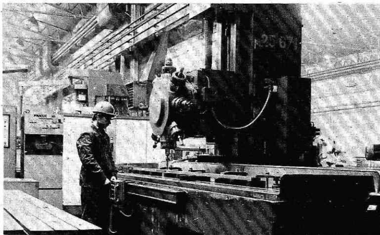
Eden od sodobnih NC vrtalnih strojev v železarni Ravne
