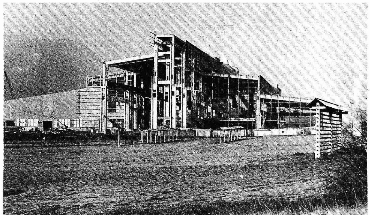
Jeklarna 2 (foto: I. Kučina)
