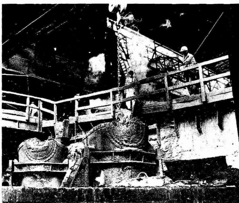
Po končanem preobodu na plavžu
