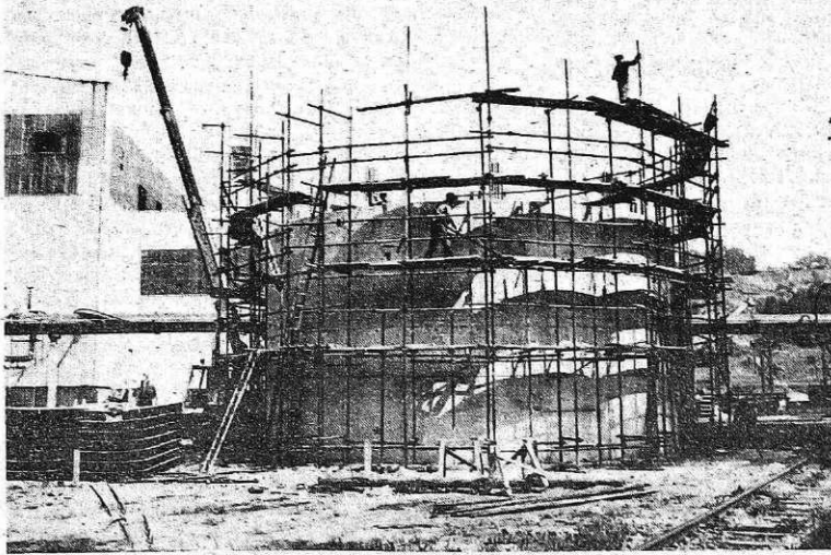
Gradnja bazena za dekarboniziranje hladilne vode za novo konti napravo v Železarni Štore
