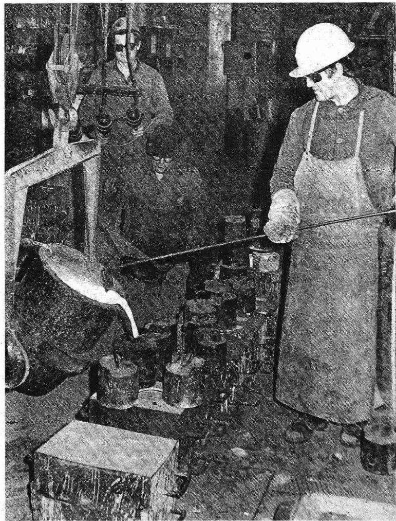
Vlivanje bronastih odlitkov v sivi livarni naše železarne (foto I. Kučina)
