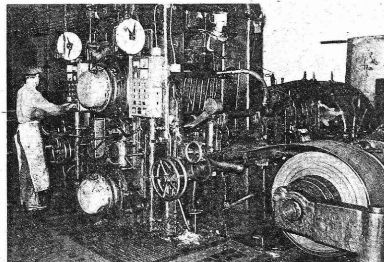
V hladni valjarni na Jesenicah (foto I. Kučina)
