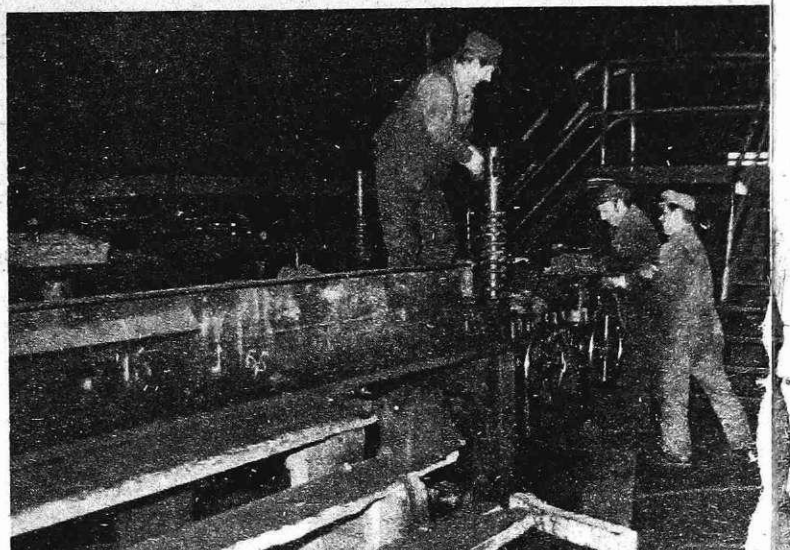
Večdnevni remont na liniji rezanja v valjarni štekel (foto I. Kučina)
