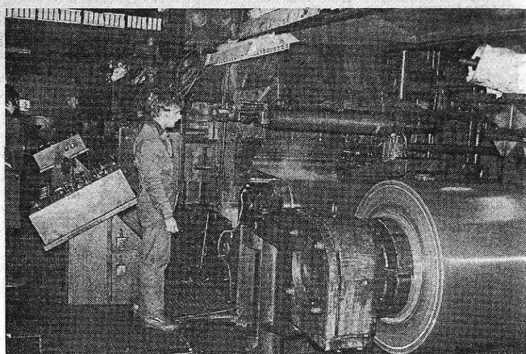
Sendzimir linija v hladni valjarni Bela (foto S. Kokalj)
