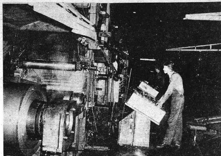
Na Sendzimir liniji (Foto S. Kokalj)
