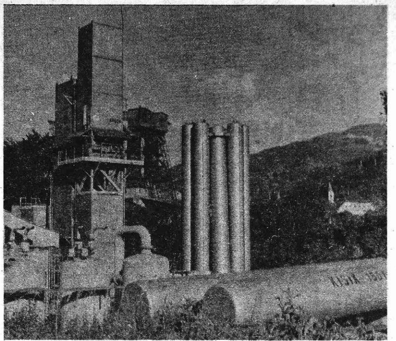
Kisikarna Sava (Foto I. Kučina)
