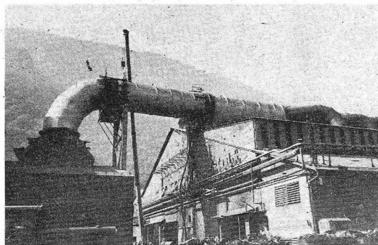
etm Nove odpraševalne naprave (Foto S. Kokalj)
