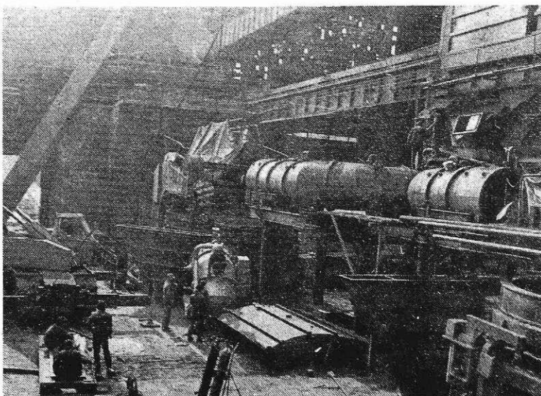
Med montažo odpraševalne naprave v elektrojeklarni (Foto S. Kokalj)
