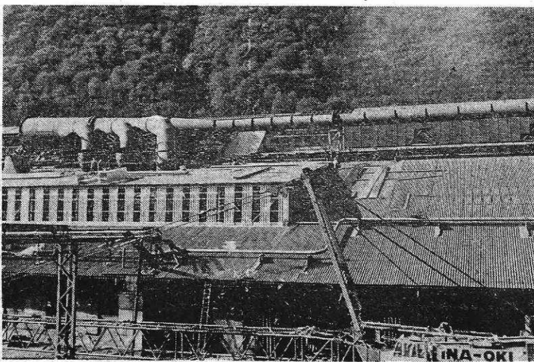
Montaža odpraševalnih naprav (Foto S. Kokalj)
