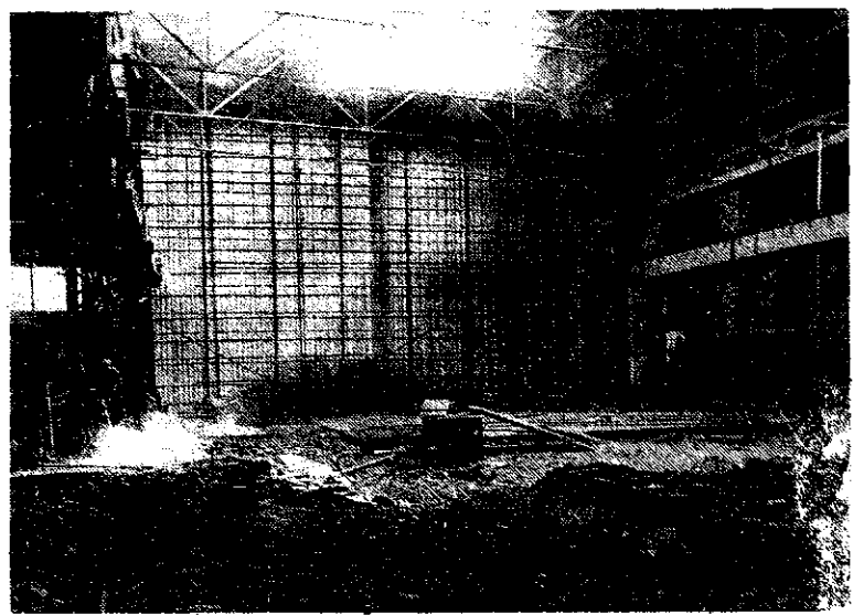
Gradnja podaljška strojne delavnice na Javorniku (Foto I. Kučina)
