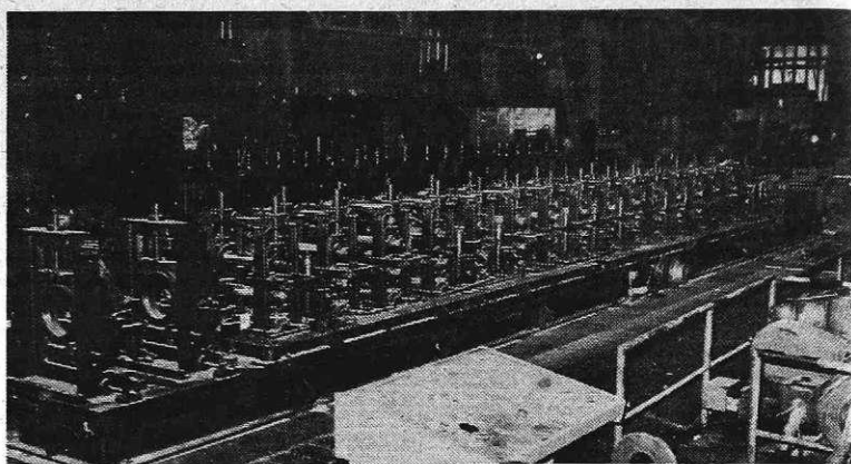
Del oblikovalne proge v profilarni na Javorniku (Foto I. Kučina)
