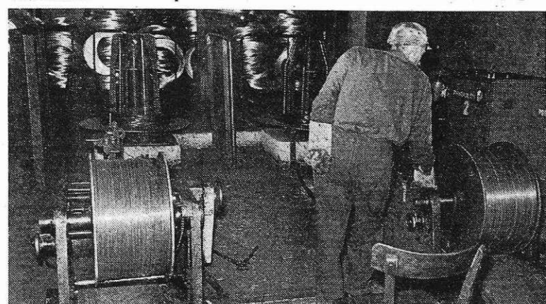
Previjalna linija v Žičarni
