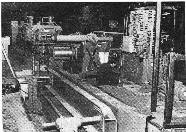
Montaža oblikovalne proge v profilarni na Javorniku (Foto I. Kučina)
