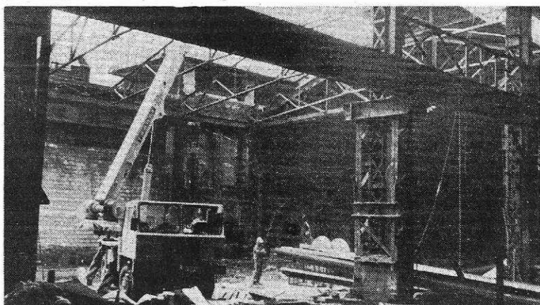
Gradnja podaljška strojnih delavnic na Javorniku (Foto I. Kučina)
