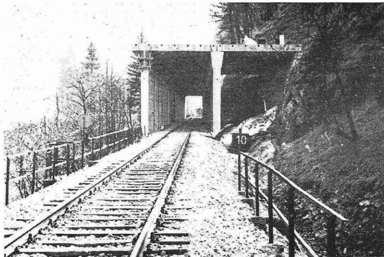
Galerija za obrambo proge pred plazovi v Soteski (Foto B. Blenkuš)
