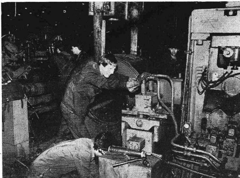
Vzdrževalci hladne valjarne Bela pri enodnevnem remontu na liniji za pravo trakov (Foto I. Kučina)
