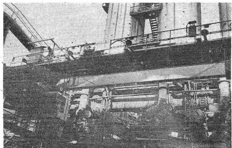
Montaža novega žerjava na Plavžu (Foto I. Kučina)
