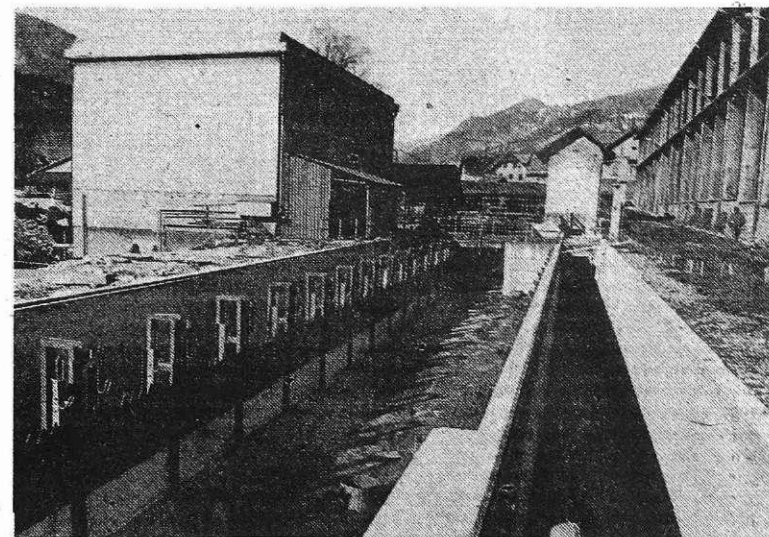
Rekonstrukcija rak na jezu za čiščenje hladilne vode za Železarno (Foto I. Kučina)
