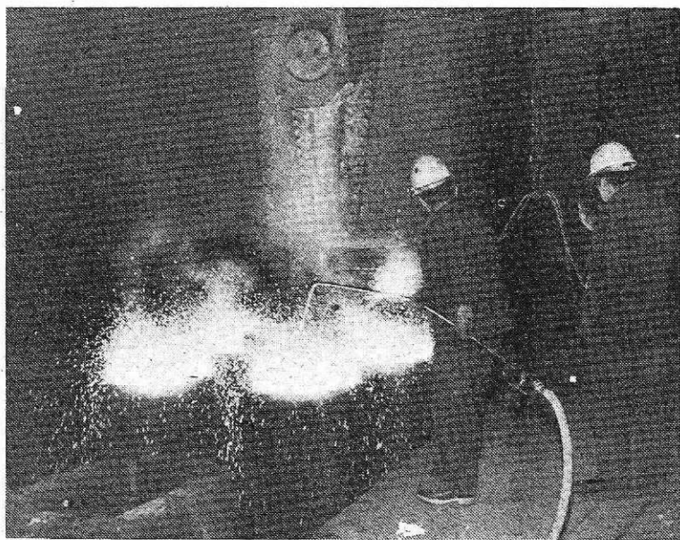
Vlivanje jekla (Foto I. Kučina)
