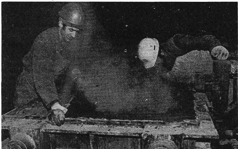
Sodelavca pri obzidavi vmesne ponvice za konti-liv (Foto I. Kučina)
