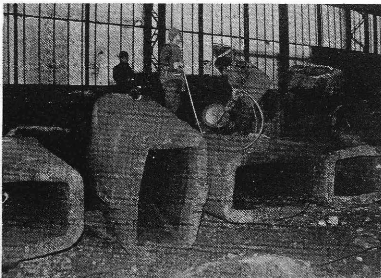
Čiščenje kobil v martinarni (Foto I. Kučina)
