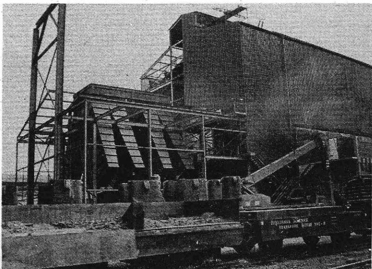
Odpraševalne naprave (Foto I. Kučina)
