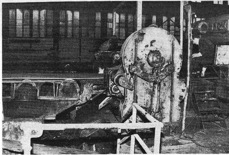
V valjarni debele pločevine (Foto I. Kučina)
