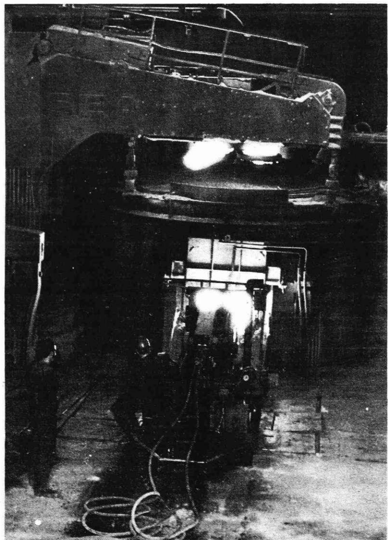
Pri ASEA električni peči
