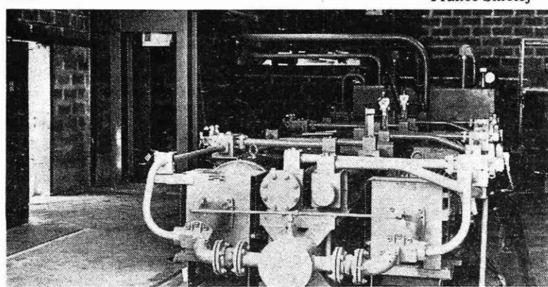
Strojnica škarij za razrez starega železa
