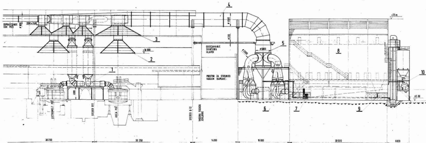
ODPRAŠEVALNA NAPRAVA ZA ELEKTROJEKLARNO
