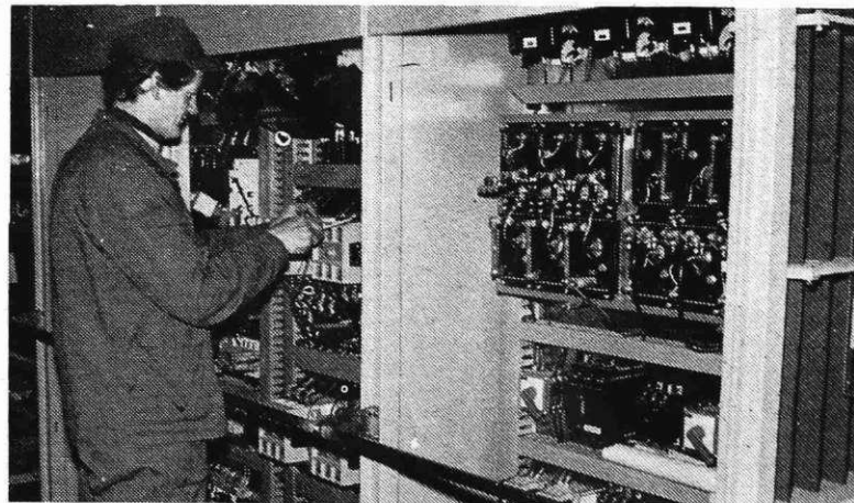
Montaža električnih stikalnih omar za konti liv
