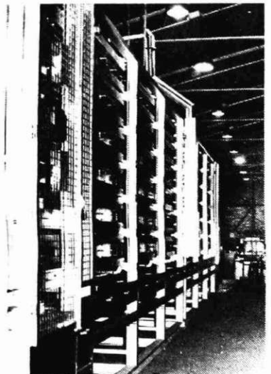
Sušilna peč za sušenje elektrod
