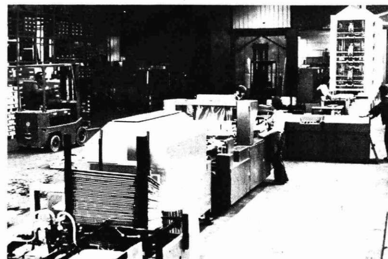
Nova moderna linija za izdelavo oplasnjenih elektrod
