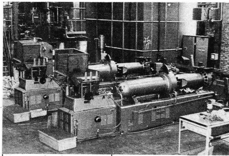
Del nove linije v TOZD Elektrode
