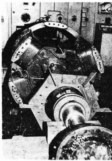
Sinhronski motor E grupe v strojnici štekel
