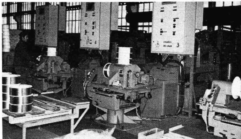
Žičarna — nova linija za VAC žico
