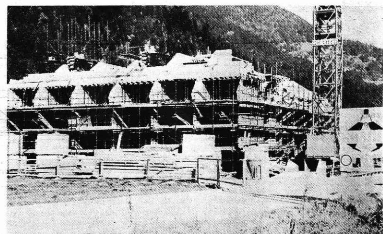
Gradnja počitniško-stanovanjske zgradbe v Kranjski gori (Foto B. Blenkuš)
