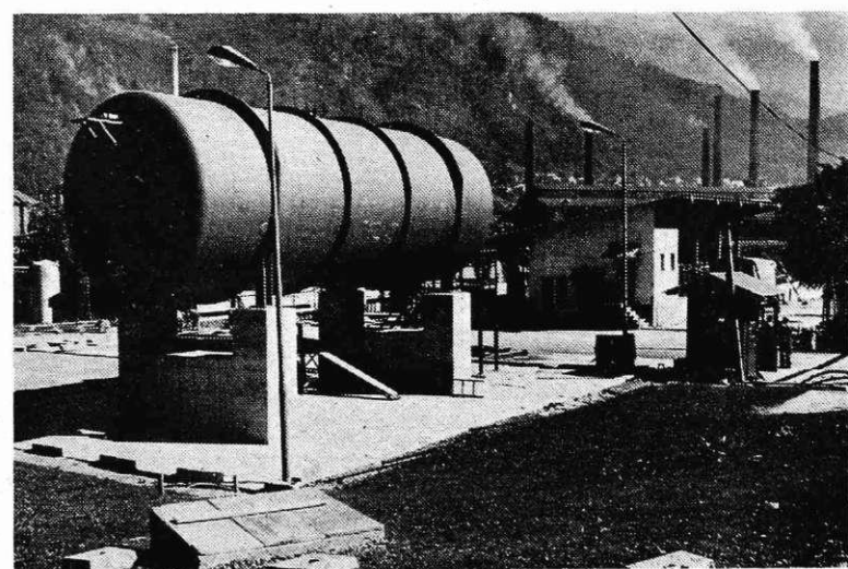
100.000 litrski tank za tekoči plin je montiran
