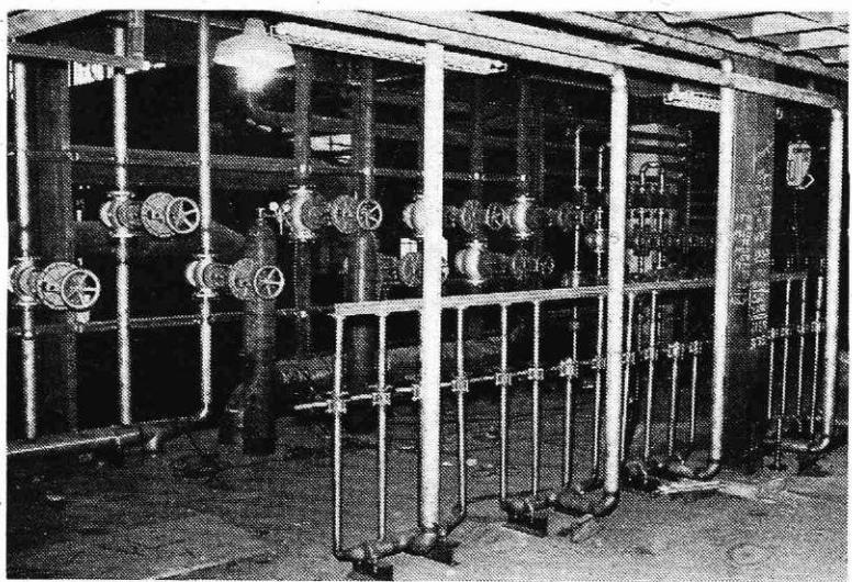
Konti liv - in stalacija za hladilno vodo
