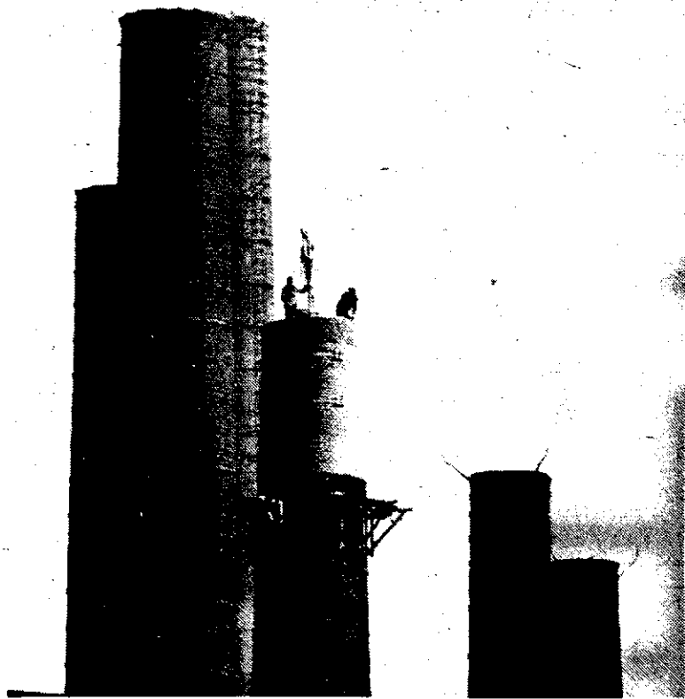
Obnova dimnika SM peči št. 3
