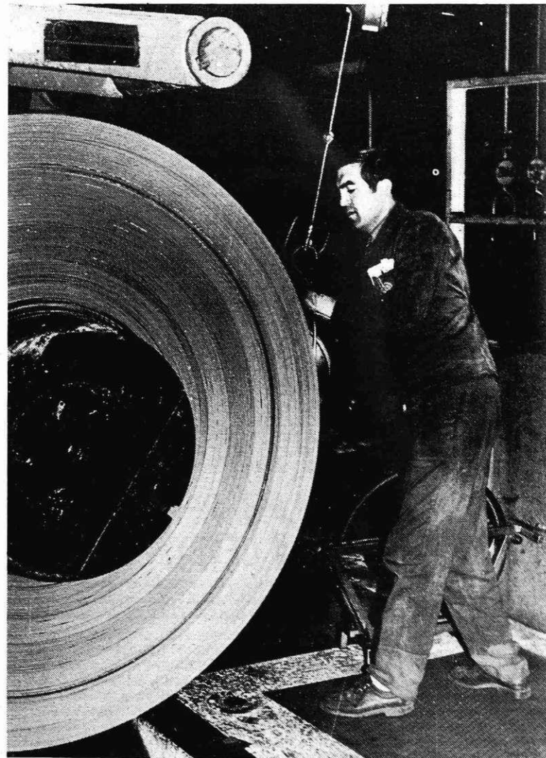
Sodelavec pri previjalni liniji v hladni valjarni Bela
