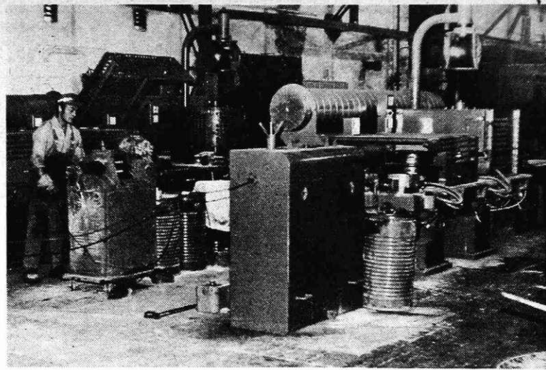
Vlečna rezalna linija v elektrodnem obratu
