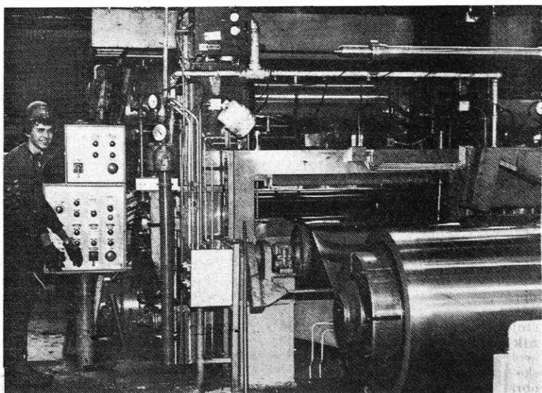
Dresirno ogrodje v hladni valjarni Bela
