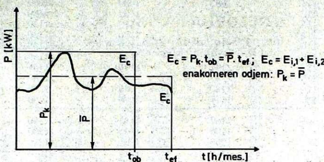
Slika št. 2: vpliv konične moči na zaračunat obseg
