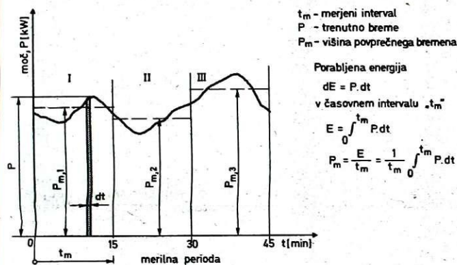
Slika št. 1: izmerjene srednje vrednosti maksimuma, kot jih beleži kWh-ura
