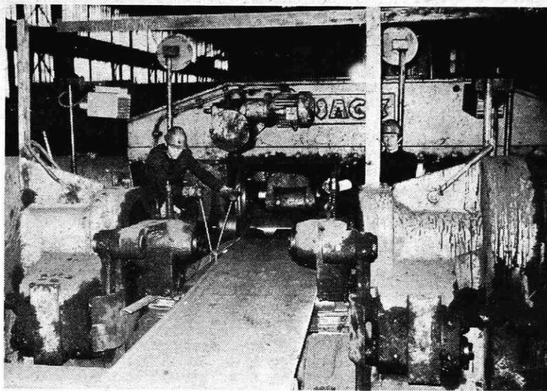
Sack škarje za razrez pločevine v valjarni debele pločevine
