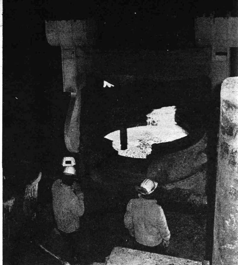
Surovo jeklo iz električne peči Lectromelt
