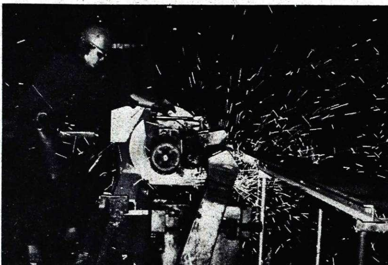
Rezalec hladno oblikovanih profilov
