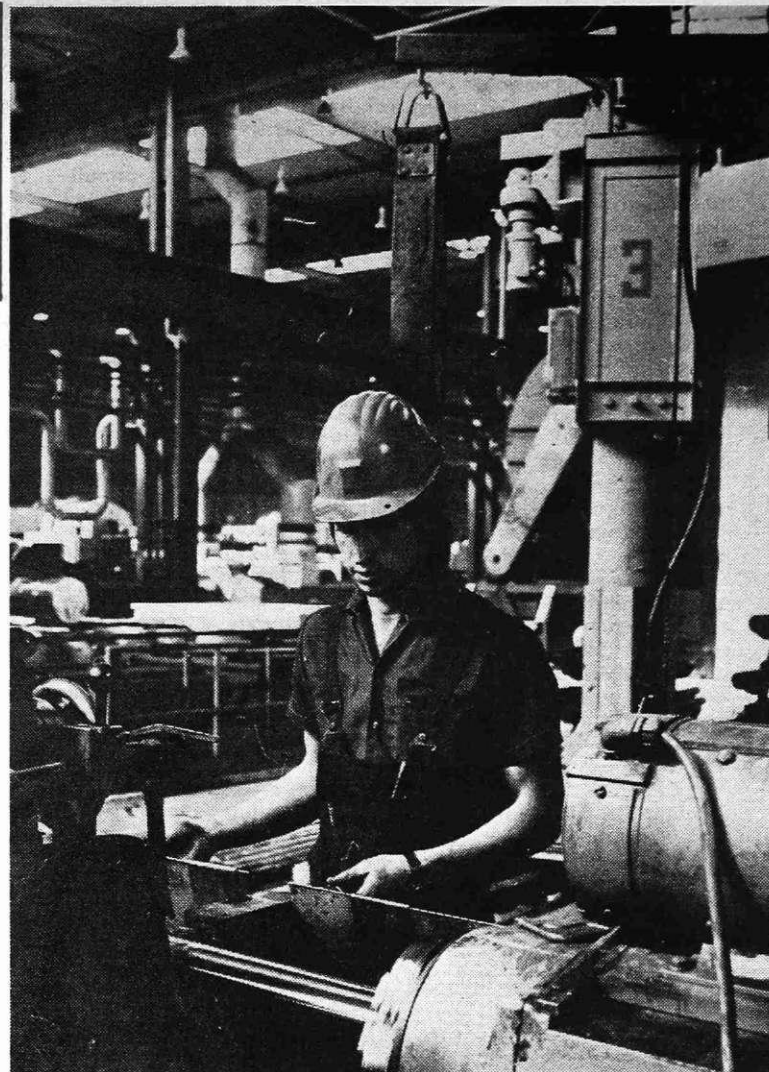
Sodelavec pri struženju Sendzimir valjev v hladni valjarni Bela
