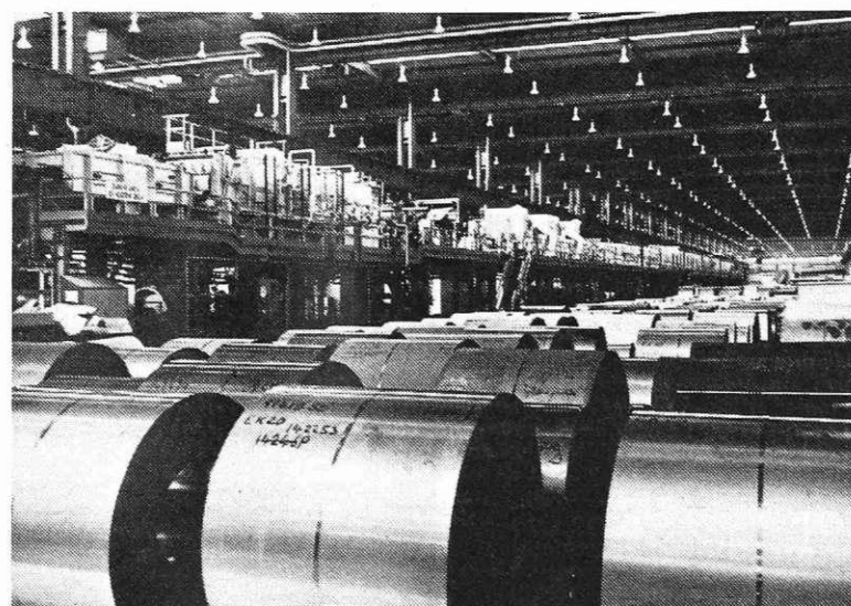
Žarilna linija za nerjavna jekla v hladni valjarni Bela
