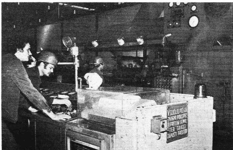
Sendzimir ogródje s komandnim pultom
