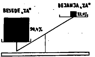
SLIKA 14: Neravnovesje med stališči o potrebnosti aktivnega kulturnega udejstvovanja in stvarno aktivnostjo občanov
