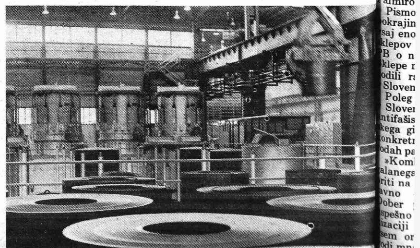
Zvonaste peči v hladni, valjarni Belp
